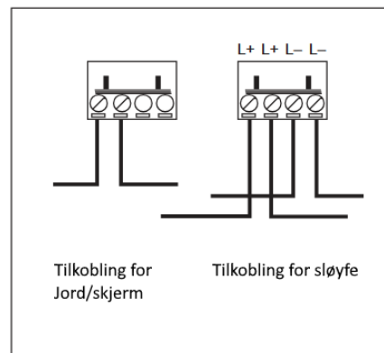
Fig 2 Koblingsklemmer
