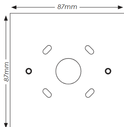
Fig 1 Bakboks
