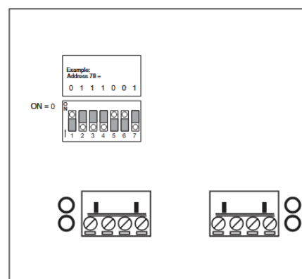
Fig 4 Koblingsklemmer og adresse satt til 78
